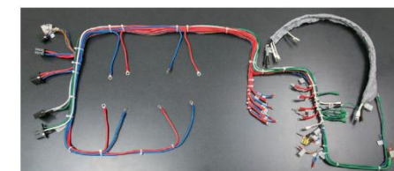
布線加工
